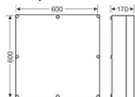
Méreterajz
